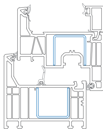
Elegante profilé non recouvert · Échelle 1:2
