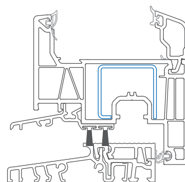
Elegante avec un seuil chaud en aluminium et une baguette arrondie · Échelle 1:2
